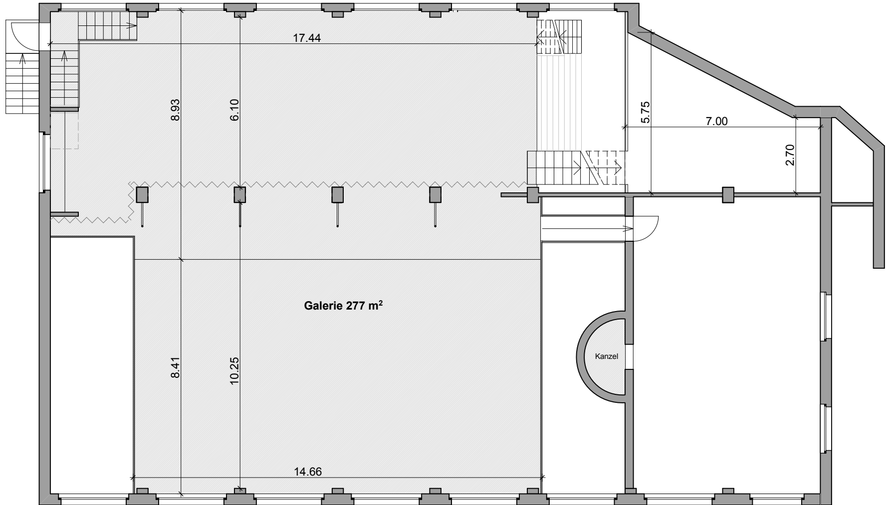
Stufenbau Eventlocation - Eventplan - Grundriss 6. Obergeschoss - Galerie
