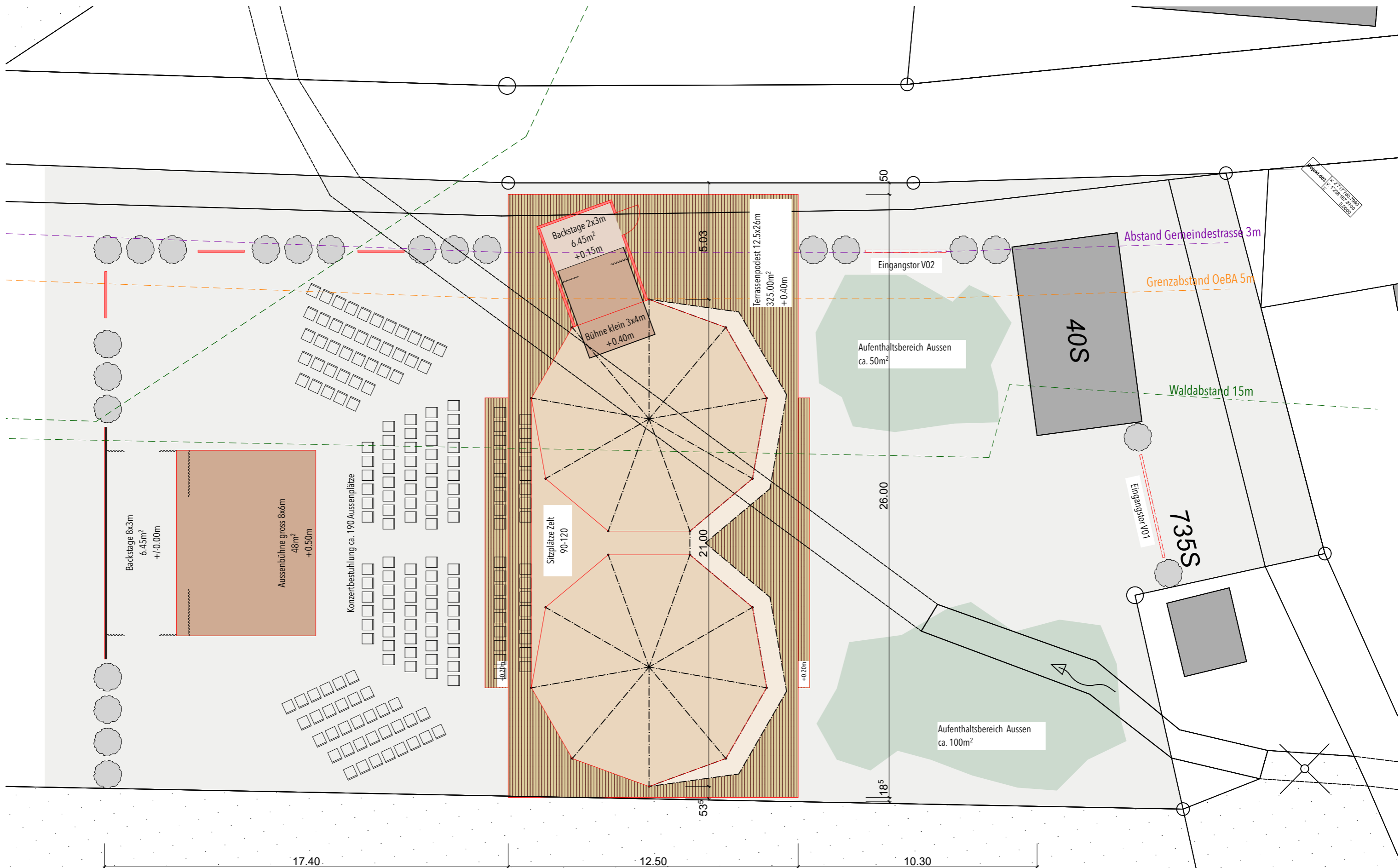
Grundriss V03 M. 1:150 ; Format A3
