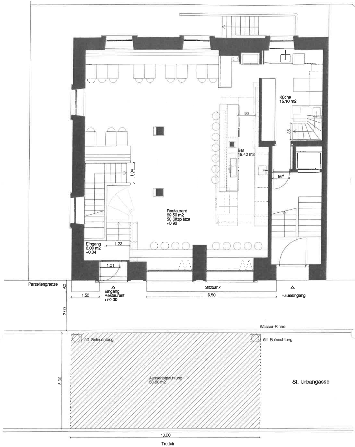
Grundriss Erdgeschoss 1:100
