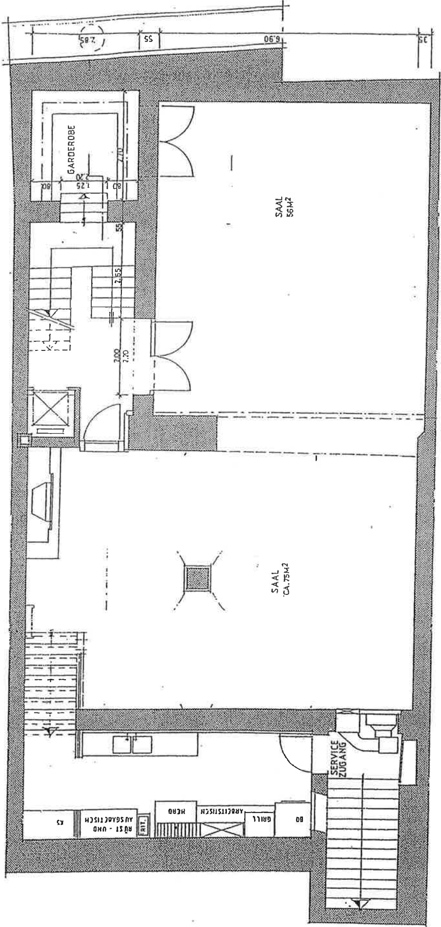
GRUNDRISS UNTERGESCHOSS
